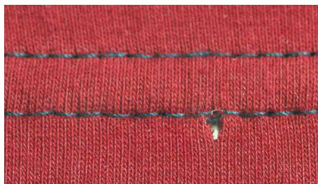
РИС 2. ПОВРЕЖДЕННЫ ПЕТЛИ - ТЕСТ ПРОДОЛЖАЕТСЯ С МЕНЬШИМ НОМЕРОМ ИГЛЫ.
